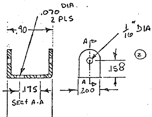
P/N M DDC 1013-0 U-BRACKET
